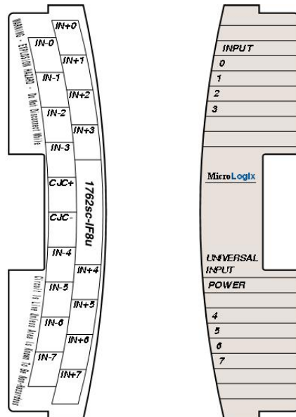
Figure 2-7. Door Label
